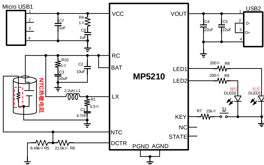
MP5210典型应用电路
